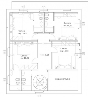
PIANO TERZO
