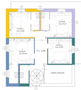
PIANO TERZO
