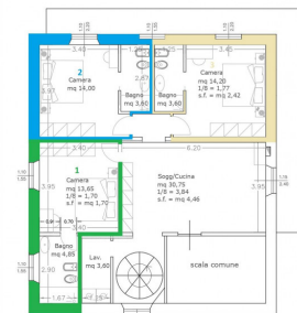
PIANO SECONDO
