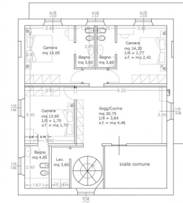
PIANO SECONDO
